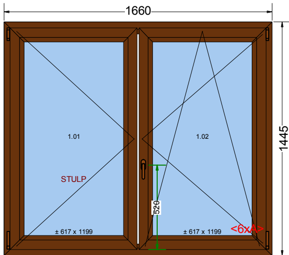
Widok wewnętrzny
