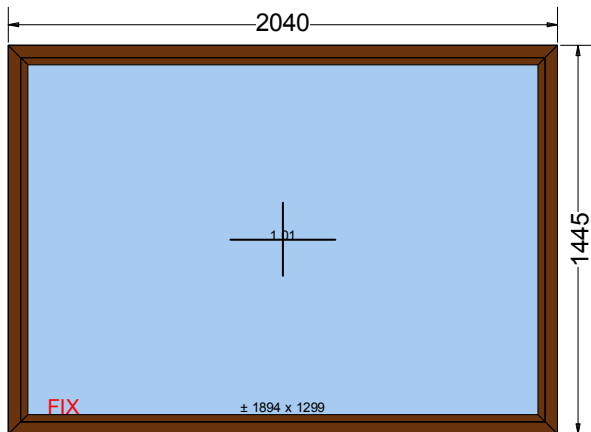
Widok wewnętrzny
