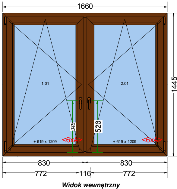
Widok wewnętrzny
