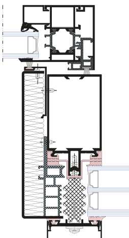
Drzwi automatyczne w fasadzie
